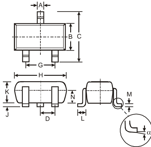
SOT523
